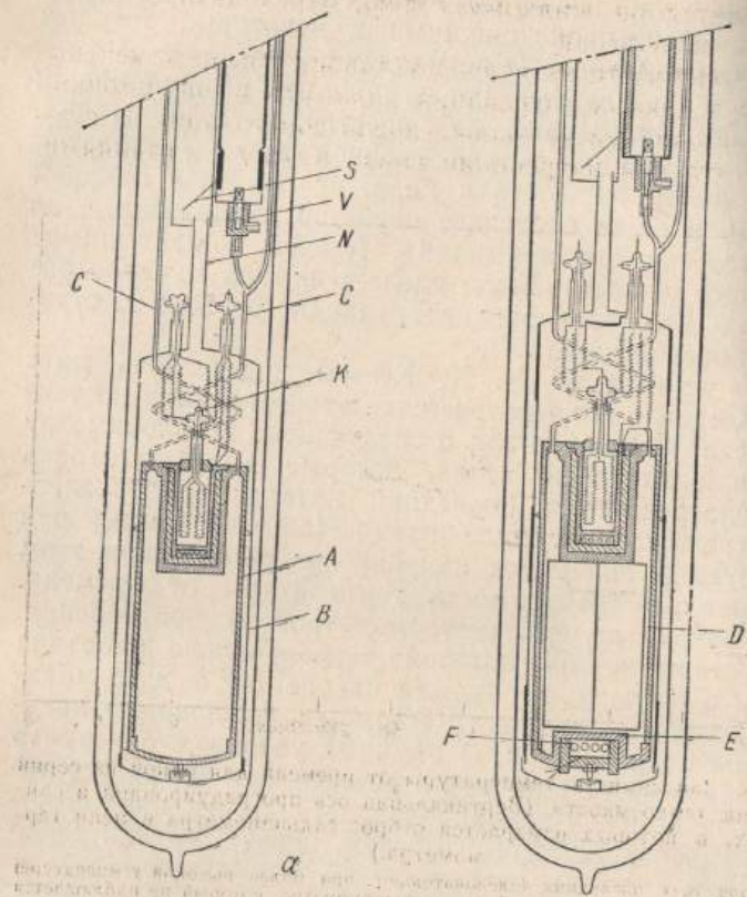
Рис. 5.4. Калориметр для жидкого гелия, использованный Кеезом и Клузиусом, а также на раннем этапе работы — Кеезом и Мисс Кеезом (а).
