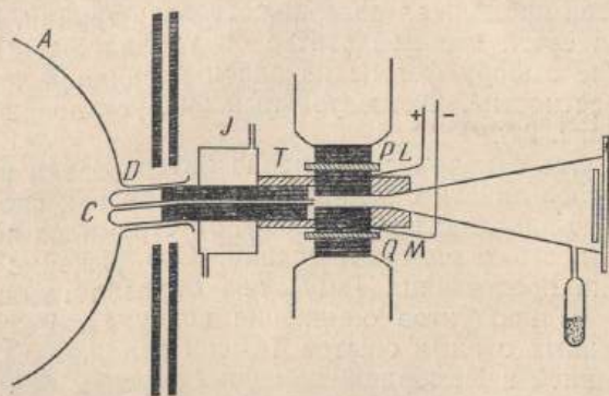
Рис. 2.8. Окончательный вид трубки, использованной Томсоном.
