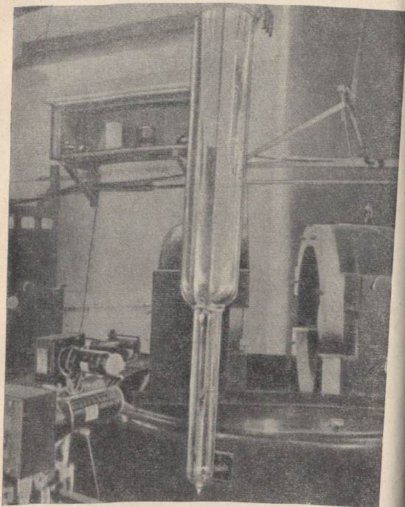
Рис. 10.2. Экспериментальная установка, на которой проводился эксперимент с поляризацией ^{60}\text{Co} .
