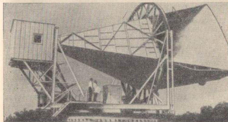
Рис. 16.2. Рупорно-отражательная антенна, использованная Пензиасом и Вильсоном [Bell Syst. Techn. Journ., 40 (1961), стр. 1097, рис. 2].
