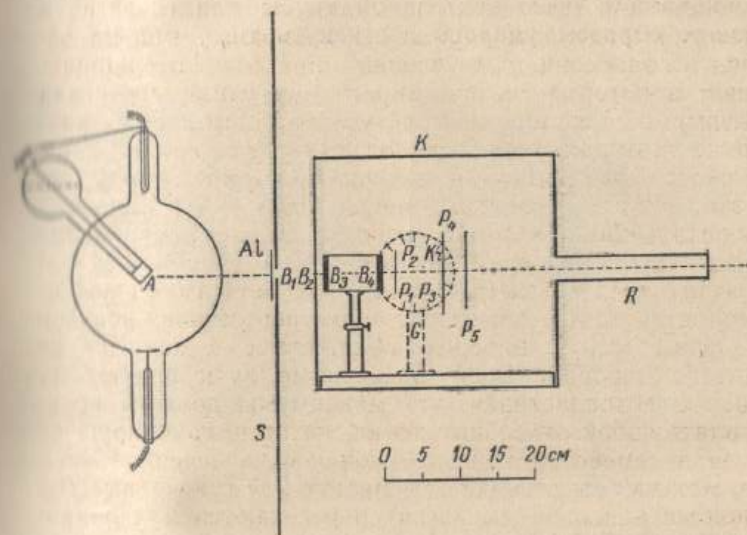
Рис. 1.1. Установка Фридриха и Кнippingа для изучения рассеяния рентгеновских лучей, проникающих сквозь кристалл [Ann. Physik, 41 (1912), стр. 979, рис. 1].
