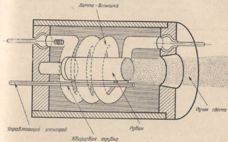
Рис. 13.4. Устройство для импульсного возбуждения рубина (размеры примерно 2 \times 1 дюйм 2 ) [ Phys. Rev. , 123 (1961), стр. 1154, рис. 7].
