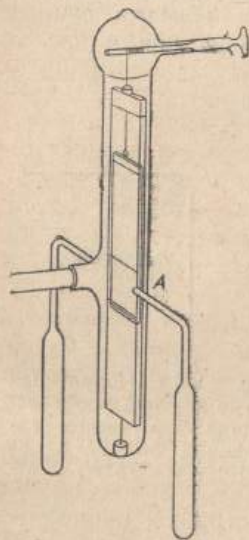
Рис. 2.7. Один из держателей фотопластин [Phil. Mag., 21 (1911), стр. 228, рис. 2].
