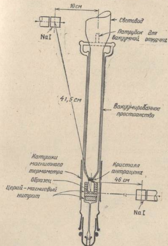
Рис. 10.1. Схематическое изображение нижней части криостата, использованного в эксперименте с поляризованным ^{60}\text{Co} [Phys. Rev., 105 (1957), стр. 1413, рис. 1].
