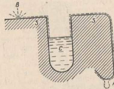
Рис. 5.17. Схема, изображающая течение пленки [Proc. Roy. Soc., Ser. A170 (1939), стр. 446, рис. 5].
