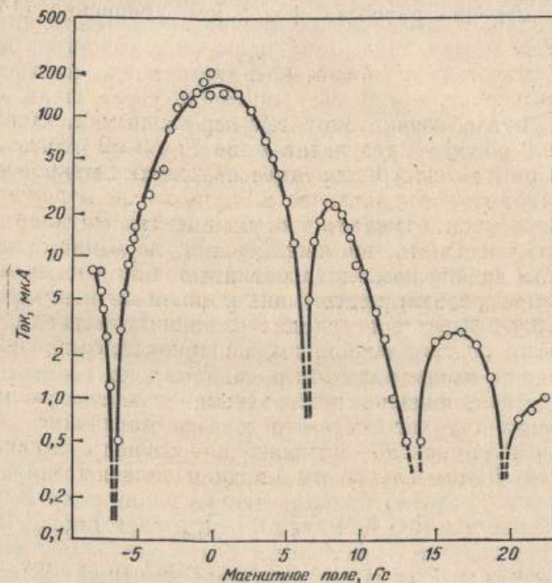
Рис. 14.7. «Зависимость максимального сверхпроводящего тока от магнитного поля для перехода свинец — диэлектрик — свинец при T = 1,3 \text{ K} ».
