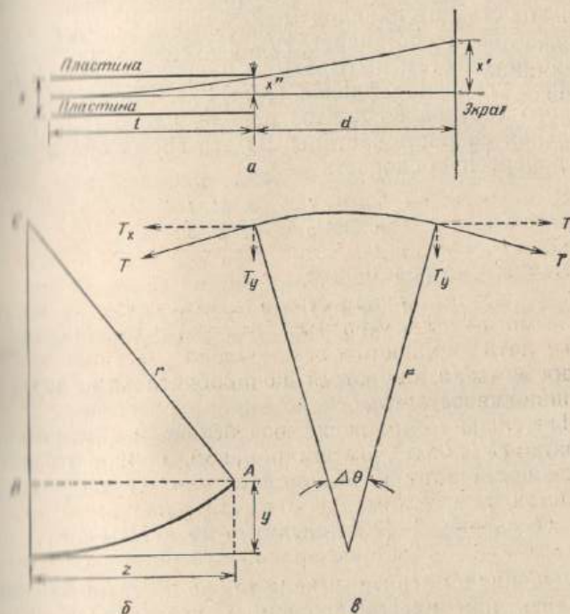
Рис. 2.2. Геометрическая иллюстрация к вычислению отклонения положительных лучей: a — в электрическом поле; b — в магнитном поле; a — провод под действием растягивающих напряжений.
