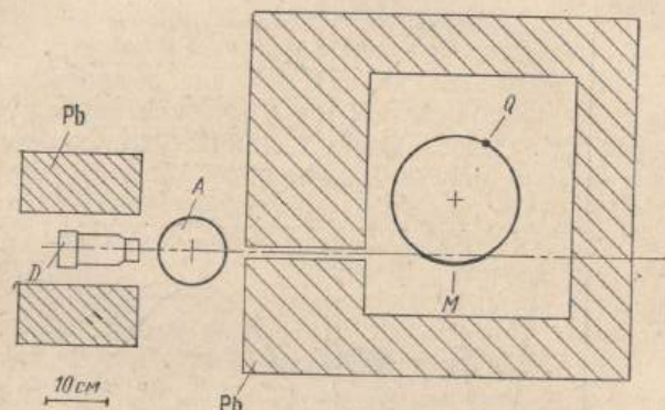
Рис. 11.5. Геометрия эксперимента.
