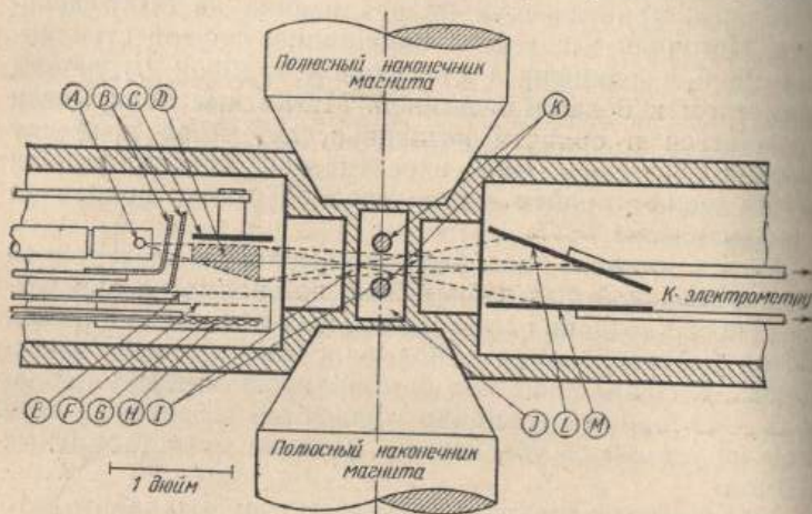
Рис. 7.4. Поперечное сечение установки.
