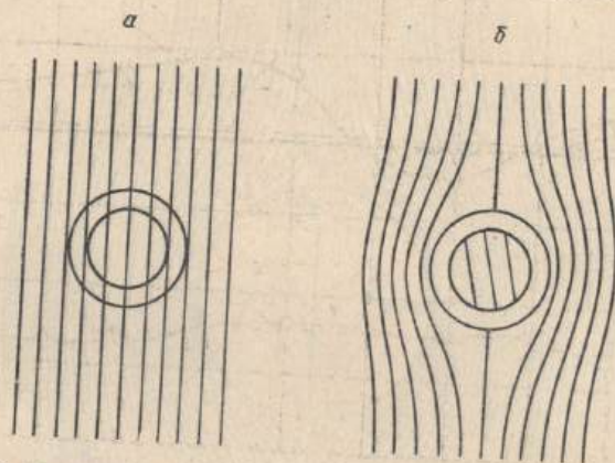
Рис. 4.10. Влияние сверхпроводящего перехода на распределение магнитного поля вблизи полого цилиндрического сверхпроводника: а — выше точки перехода; б — ниже точки перехода [Z. ges. Kälte-Ind., 11 (1934), стр. 127, рис. 4],
