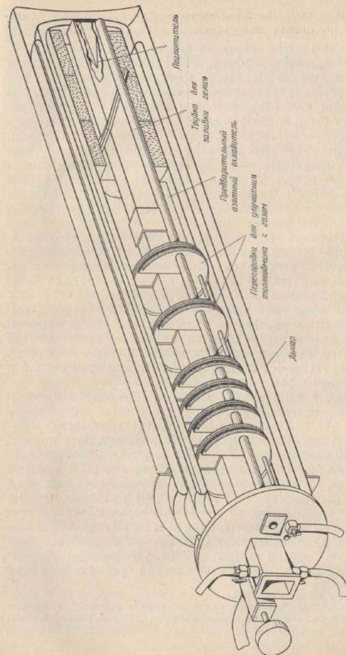
Рис. 16.4. Изометрическая проекция источника опорного сигнала, смонтированного в дьюаре. В рабочем положении прибор стоит вертикально, закрытым концом вниз [Rev. Sci. Instr., 36 (1965), стр. 69, рис. 1].
