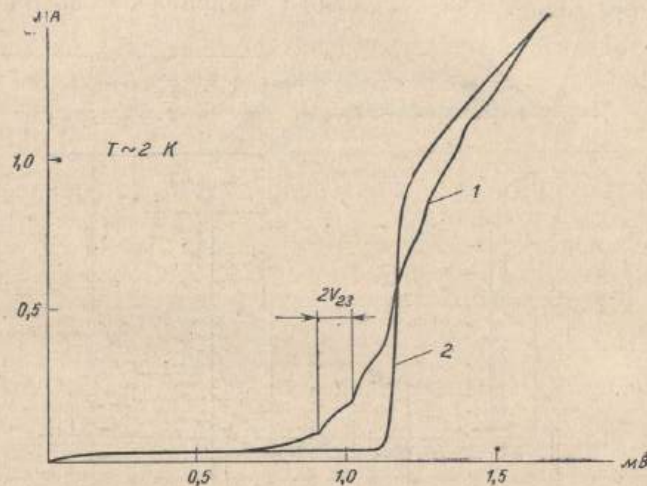
Рис. 14.11. Вольт-амперные характеристики детектирующего туннельного перехода в эксперименте Живера для случаев, когда напряжение на генерирующем переходе приложено (1) и когда оно отсутствует (2) [Phys. Rev. Lett., 14 (1965), стр. 905, рис. 2].
