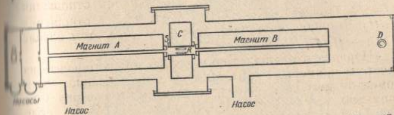
Рис. 6.2. Конструктивная схема реальной установки [Phys. Rev., 55 (1939), стр. 529, рис. 2].
