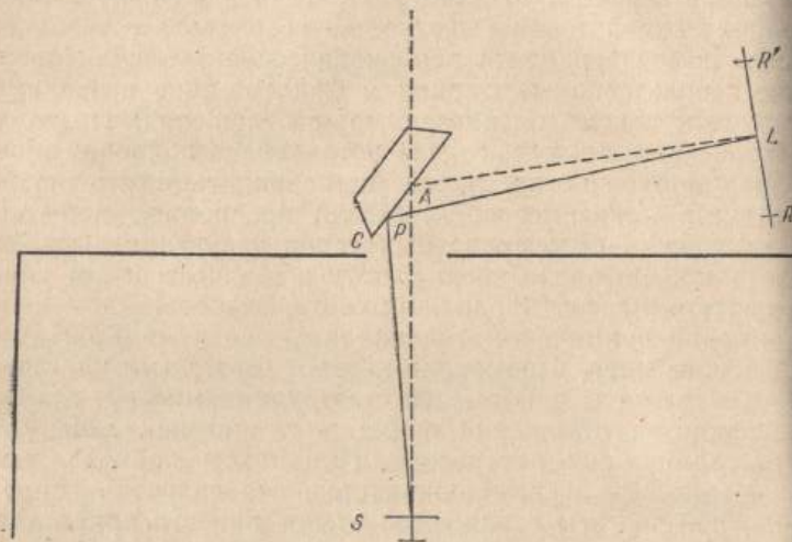
Рис. 3.1. Схема расположения кристалла, источника со щелью и фотопластины в установке Мозли [Phil. Mag., 26 (1913), стр. 1025, рис. 1].
