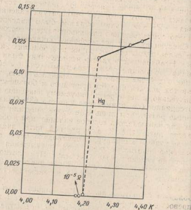
Рис. 4.5. Зависимость сопротивления образца ртути от температуры [Comm. Phys. Lab. Univ. Leiden, № 124 (1912), стр. 23, рис. без номера].
