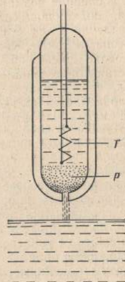
Рис. 5.19. Прибор для демонстрации механического эффекта, обратного эффекту фонтанирования [Nature, 143 (1939), стр. 719, рис. 2].
