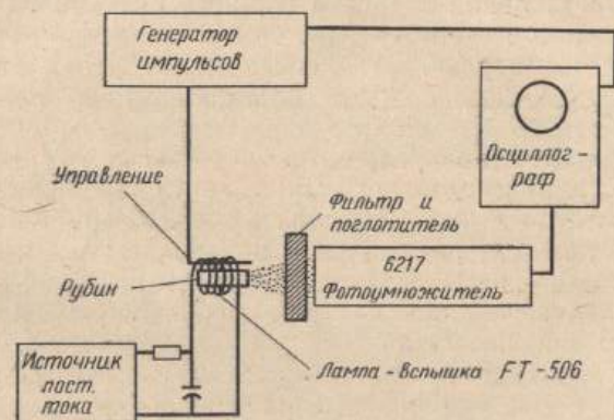
Рис. 13.5. Блок-схема экспериментальной установки для наблюдения индуцированного излучения в рубине [Phys. Rev., 123 (1961), стр. 1154, рис. 8].
