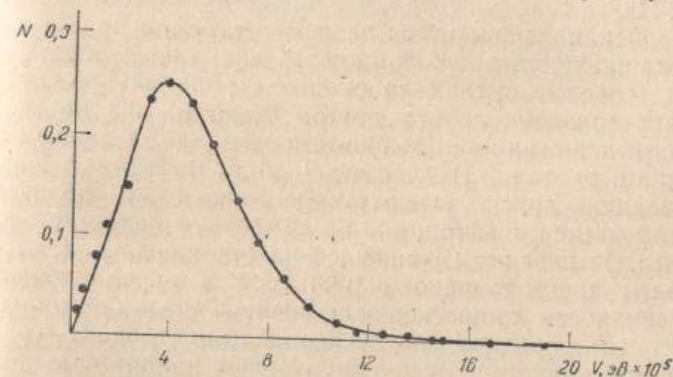
Рис. 12.1. Энергетический спектр \beta -излучения, испускаемого \text{RaE} (^{210}\text{Bi}) [ Phys. Rev. , 48 (1935), стр. 394, рис. 5].
