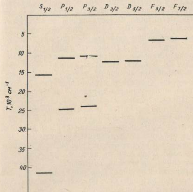
Рис. 15.1. Некоторые энергетические уровни атома натрия.
