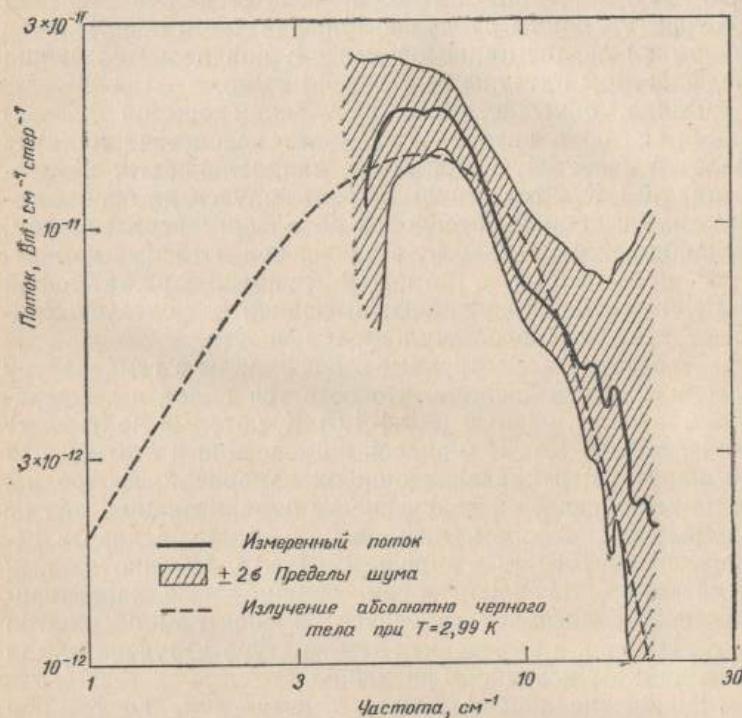
Рис. 16.5. Сравнение спектра космического фонового излучения, измеренного Вуди и др., со спектром абсолютно черного тела при температуре 2,99 К. ( \sigma — стандартное отклонение) [ Phys. Rev. Lett. , 34 (1975), стр. 1038, рис. 2].
