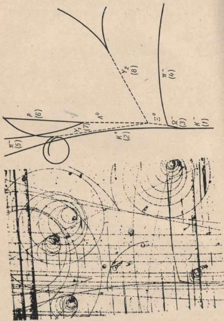
Рис. 15.6. Фотография и диаграмма процесса распада Q^- -гиперона [Phys. Rev. Lett., 12 (1964), стр. 205, рис. 2].
