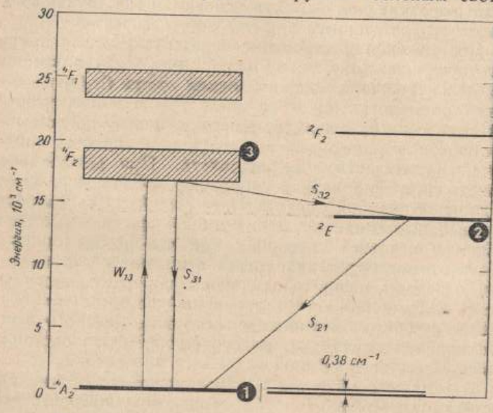
Рис. 13.3. Схема энергетических уровней в рубине. Заштрихованные полосы обозначают широкие зоны энергии. Символы, нанесенные рядом с уровнями, описывают определенные свойства симметрии этих уровней [Phys. Rev. Lett., 4 (1960), стр. 564, рис. 1].
