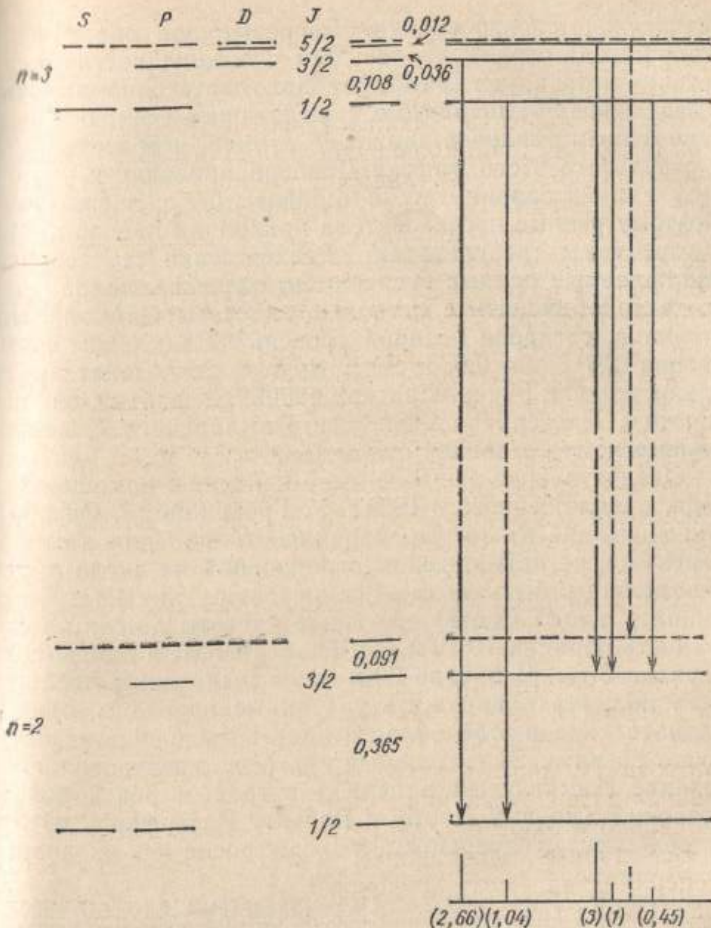
Рис. 7.1. Структура уровней энергии водорода с n = 2 и n = 3 .
