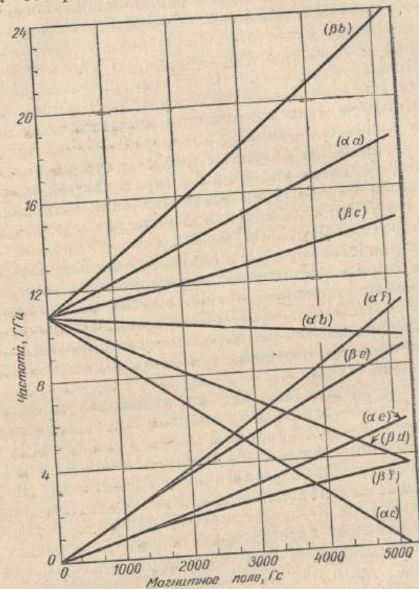
Рис. 7.3. Зависимость от магнитного поля резонансных частот, ожидаемых на основании теории Дирака для переходов между состояниями водорода с n=2 . Пары букв обозначают переходы между соответствующими состояниями, обозначенными так же, как на рис. 7.2 [Phys. Rev., 79 (1950), стр. 560, рис. 13].
