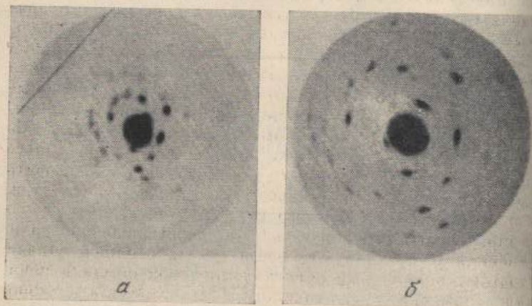
Рис. 1.2. Две картины рассеяния, полученные при первой экспозиции: а — на пластине P_4 (см. рис. 1.1); б — на пластинке P_5 [Ann. Physik, 41 (1912), лист I, рис. 2 и 1 соотв.].
