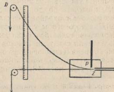
Рис. 2.3. Использование гибкого провода для определения распределения магнитного поля [Phil. Mag., 13 (1907), стр. 565, рис. 3]
