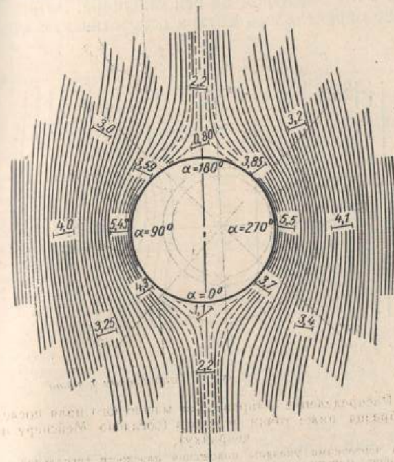
Рис. 4.9. Распределение силовых линий поля вокруг монокристалла олова в сверхпроводящем состоянии (черточки — метки направлений, перенесенные с рис. 4.8) [Physik Z., 35 (1933), стр. 934, рис. 7].
