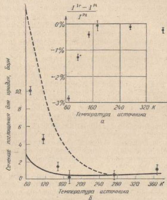
Рис. 11.3. Изменение относительной разности интенсивностей \gamma -излучения после поглощения в иридии и платине в зависимости от температуры источника (а). (Температура поглотителей 88 К.) Сечение резонансного поглощения \gamma -излучения ^{191}\text{Ir} в зависимости от температуры (б), полученное на основании данных, приведенных в части (а) [Z. Physik, 151 (1958), стр. 140, рис. 8].
