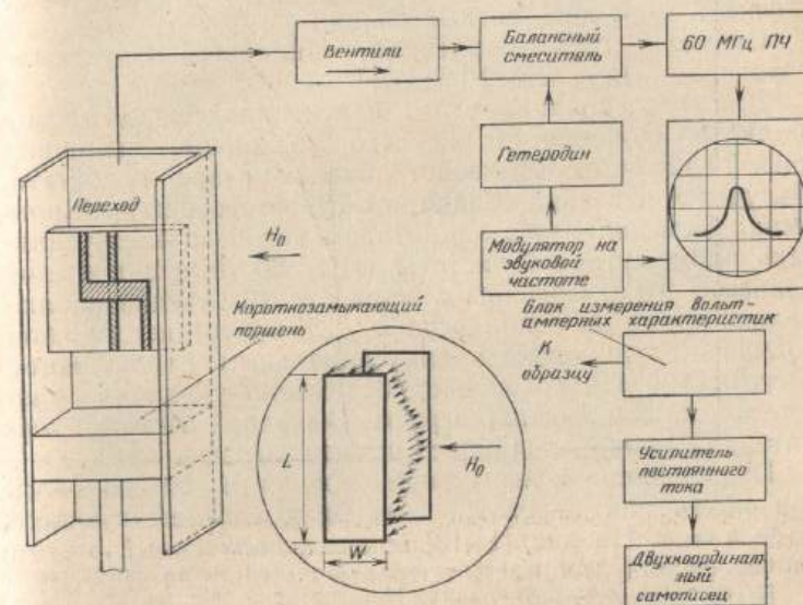
Рис. 14.12. Схема установки, использованной Лангенбергом, Скалапино, Тэйлором и Экком для непосредственного наблюдения нестационарного эффекта Джозефсона [Phys. Rev. Lett., 15 (1965), стр. 294, рис. 1].
