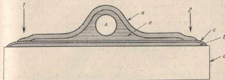
Рис. 14.14. «Поперечное сечение пары переходов Джозефсона, напыленных на кварцевую подложку (d).
