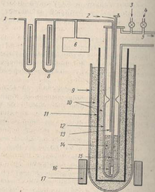
Рис. 14.2. Схема установки, использованной Живером с сотрудниками при изучении туннелирования электронов.
