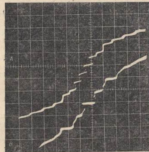
Рис. 14.9. Ступеньки, возникающие на вольт-амперных характеристиках туннельных переходов под действием СВЧ-излучения.
