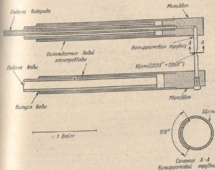
Рис. 7.5. Устройство водородного диссоциатора [Phys. Rev., 79 (1950), стр. 564, рис. 20].
