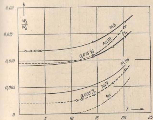
Рис. 4.3. Сопротивление двух образцов из платины и двух — из золота (тонкие пунктирные линии для образцов из золота — экстраполяция) [Commun. Phys. Lab. Univ. Leiden, № 119 (1911), лист III, рис. 3].
