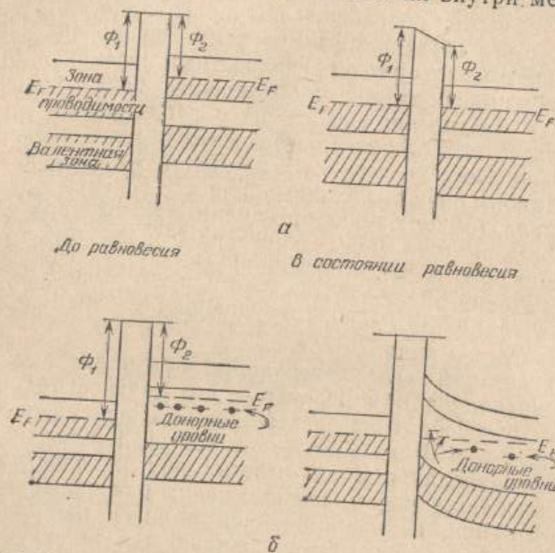
Рис. 9.2. Схема уровней энергии при контакте между двумя металлами (а) и между металлом и примесным полупроводником (б) ( \Phi — работа выхода).
