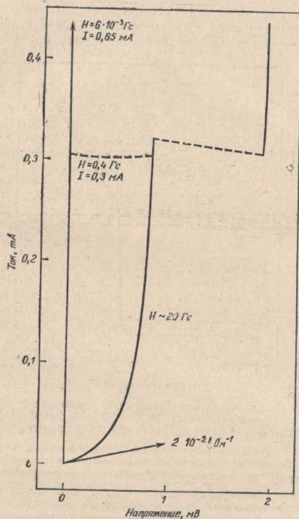
Рис. 14.6. Начальный участок зависимости, приведенной на рис. 14.5, в увеличенном масштабе вместе с вольт-амперной характеристикой перехода в поле \sim 20 Гс [Phys. Rev. Lett., 10 (1963), стр. 230, рис. 2].
