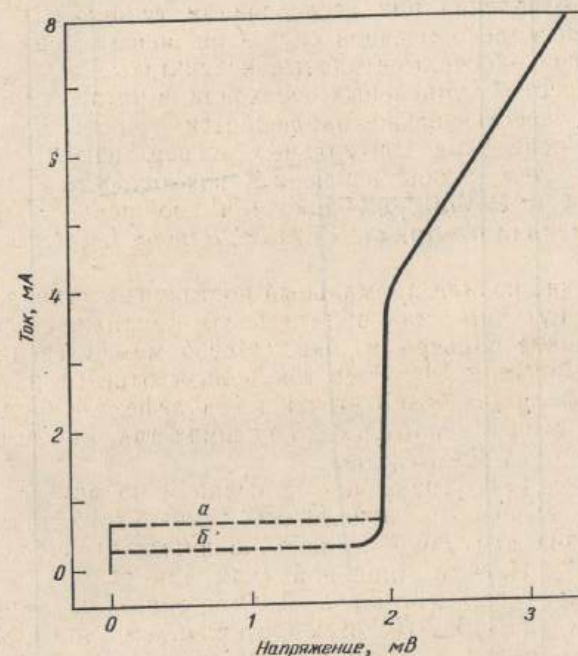
Рис. 14.5. Вольт-амперная характеристика туннельного перехода олово — окись олова — свинец при T \sim 1,5 \text{ К} в [магнитном] поле 6 \times 10^{-3} \text{ Гс} (а) и 0,4 \text{ Гс} (б) [ Phys. Rev. Lett. , 10 (1963), стр. 230, рис. 1].
