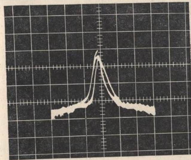
Рис. 14.13. Сигнал, наблюдавшийся Лангенбергом, Скалапино, Тэйлором и Экком при изучении перехода Джозефсона, излучающего на частоте 9,2 ГГц.
