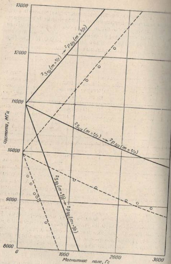
Рис. 7.7. Сравнение экспериментальных значений резонансных магнитных полей для различных частот (отмечены кружками) и значений, предсказанных теорией Дирака (сплошные линии). Те же значения, вычисленные с учетом сдвига уровня 2^2S_{1/2} вверх на 1000 МГц, обозначены пунктирными линиями. Этот график охватывает лишь малую область значений частот и магнитных полей, измеренную экспериментально, однако полный график не позволил бы рассмотреть мелкие детали; остальная часть графика тоже обнаруживает сдвиг, полностью соответствующий сдвигу на 1000 МГц [Phys. Rev., 72 (1947), стр. 242, рис. 2].
