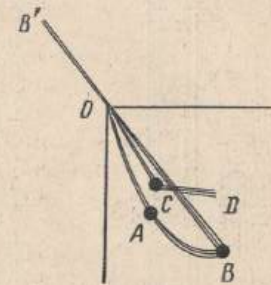
Рис. 2.6. Полученная позже картина фосфоресценции при низком давлении [Phil. Mag., 20 (1910), стр. 754, рис. 3].
