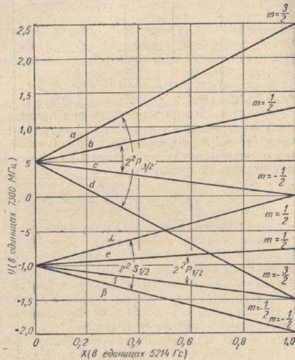
Рис. 7.2. Зеемановское расщепление уровней с n=2 в водороде. По вертикальной оси отложена энергия в единицах 2^2(E_+ - E_-) (соответствующая этой единице энергии частота равна 7300 МГц). E_+ и E_- — энергии верхнего ( 2^2P_{1/2} ) и нижнего ( 2^2S_{1/2} ) состояний в отсутствие внешнего магнитного поля. За нуль отсчета выбран «центр тяжести» этих состояний 1/2(2E_+ + E_-) . По горизонтальной оси отложено значение магнитного поля в единицах 2(E_+ - E_-)/3\mu_0 = 5214 Гс, где \mu_0 = eh/mc — магнетон Бора [Phys. Rev., 79 (1950), стр. 559, рис. 12].
