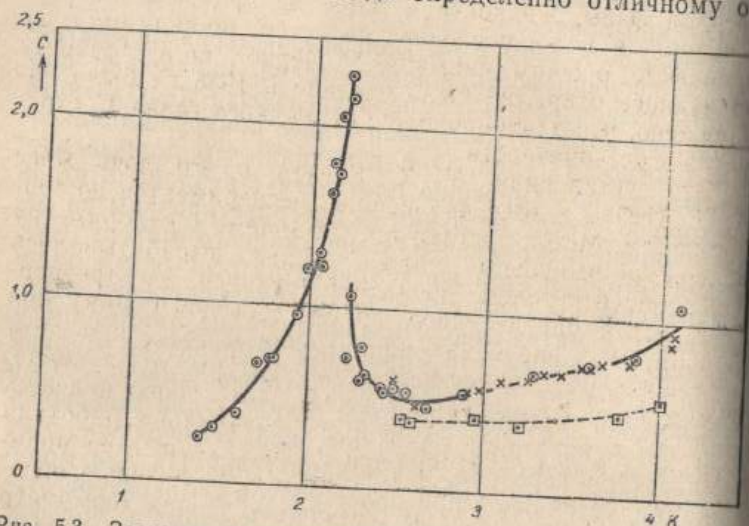
Рис. 5.3. Зависимость теплоемкости жидкого гелия (кал/г·К) от температуры.
