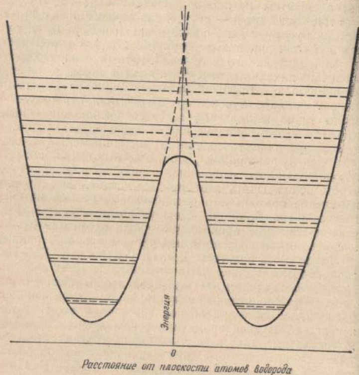
Рис. 13.1. Схема зависимости потенциальной энергии атома азота от его расположения в молекуле аммиака и характерные уровни энергии. Сплошная линия соответствует реальной ситуации, пунктирная — воображаемому случаю, когда атом азота расположен лишь по одну сторону от плоскости атомов водорода.
