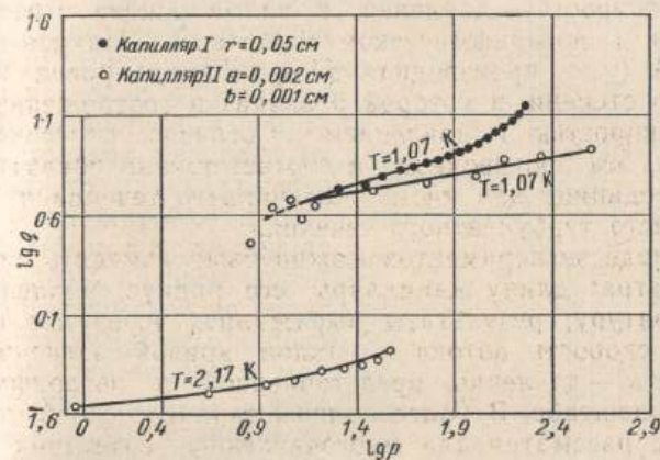
Рис. 5.7. Зависимость (в логарифмическом масштабе) скорости (см/с) от давления (дина/см²) при течении жидкого гелия II в капиллярах [Nature, 141 (1938), стр. 75, рис. без номера].
