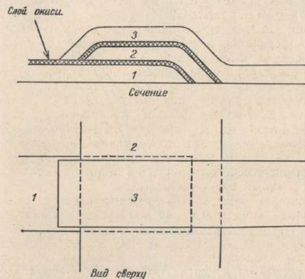
Рис. 14.10. Схематическое изображение туннельной структуры, использованной Живером при наблюдении нестационарного эффекта Джозефсона.
