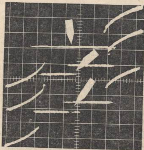
Рис. 14.8. Влияние СВЧ-излучения на вольт-амперную характеристику туннельного перехода.
