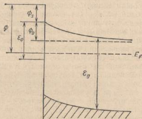
Рис. 9.3. Схема уровней энергии для состояний на и вблизи поверхности полупроводника, учитывающая поверхностные состояния [Phys. Rev., 71 (1947), стр. 722, рис. 3].
