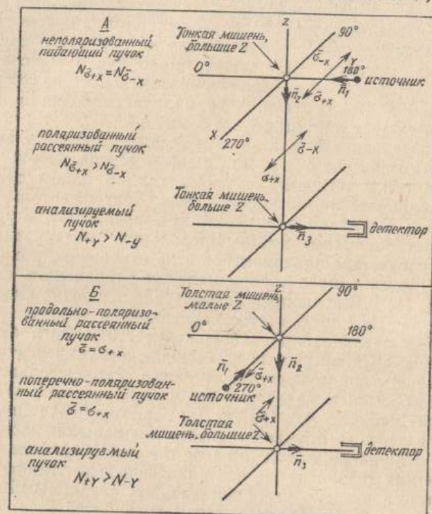
Рис. 10.8. Геометрия опыта для наблюдения двойного рассеяния (источник поворачивается, детектор неподвижен).
