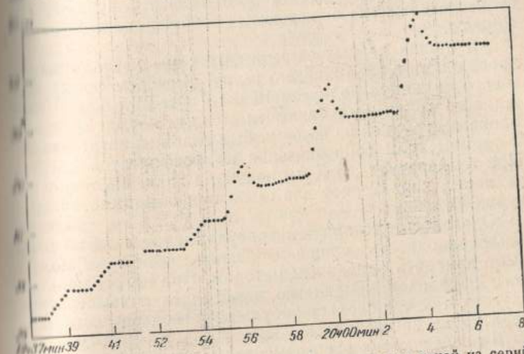
Рис. 5.5. Зависимость температуры от времени для одной из серий измерения теплоемкости. (Вертикальная ось проградуирована в сантиметрах, в которых измеряется отброс гальванометра в цепи термометра.)
