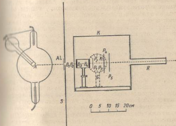
Рис. 1.1. Установка Фридриха и Книппинга для изучения рассеяния рентгеновских лучей, проникающих сквозь кристалл [Ann. Physik, 41 (1912), стр. 979, рис. 1].
