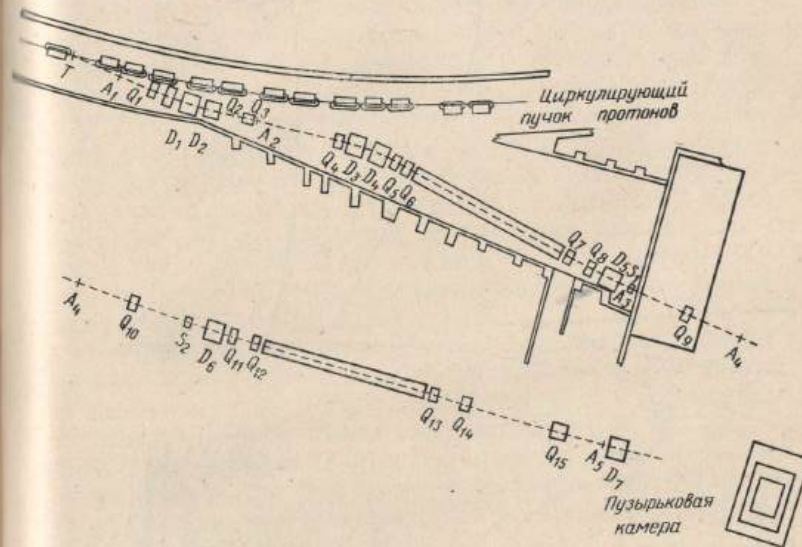
Рис 15.5. Схема прохождения пучков частиц в эксперименте по обнаружению \Omega^- -гиперона (из-за недостатка места разбита на две части).
