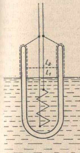
Рис. 5.18. Прибор для демонстрации течения жидкого гелия II под действием градиента температуры [Nature, 143 (1939), стр. 719, рис. 1].
