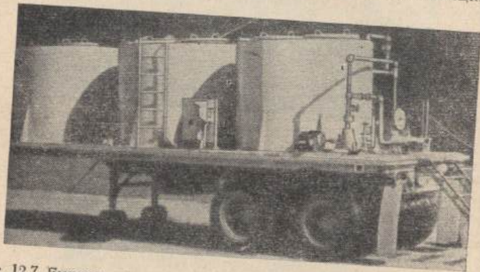
Рис. 12.7. Емкости для хранения жидких материалов [Смитсониевский отчет за 1964 г., Смитсониевский институт, Вашингтон, лист 3, рис. 1].
