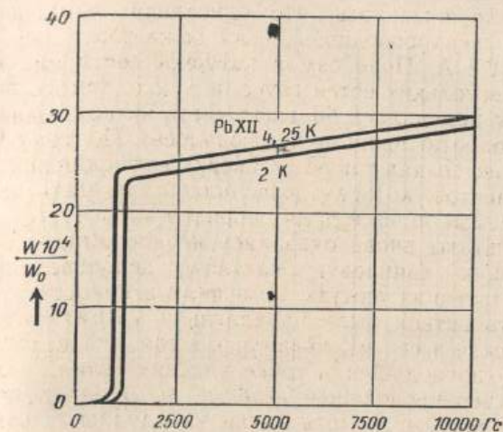
Рис. 4.6. Зависимость сопротивления катушки из свинца от приложенного магнитного поля при двух значениях температуры [Compt. rend. Phys. Lab. Univ. Leiden, № 139 (1913), стр. 67, рис. 1].
