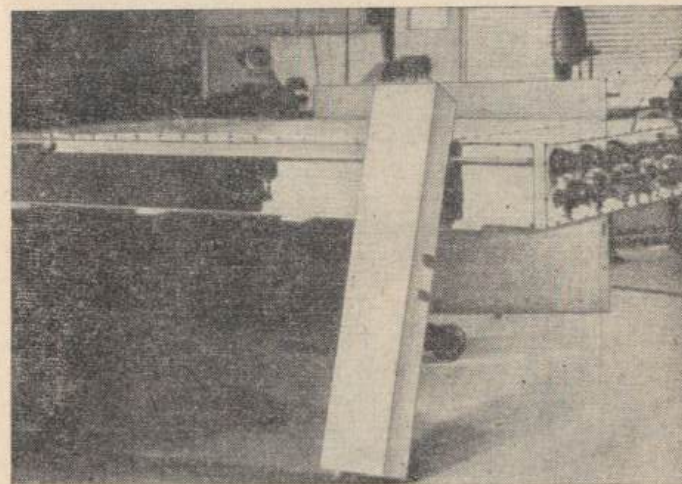
Рис. 12.4. Одна из мишеней, которая использовалась для проверки и калибровки (поэтому на ней можно увидеть цоколи фотоумножителей) [Смитсоновский отчет за 1964 г., Смитсоновский институт, Вашингтон, 1965, лист 2, рис. 1].
